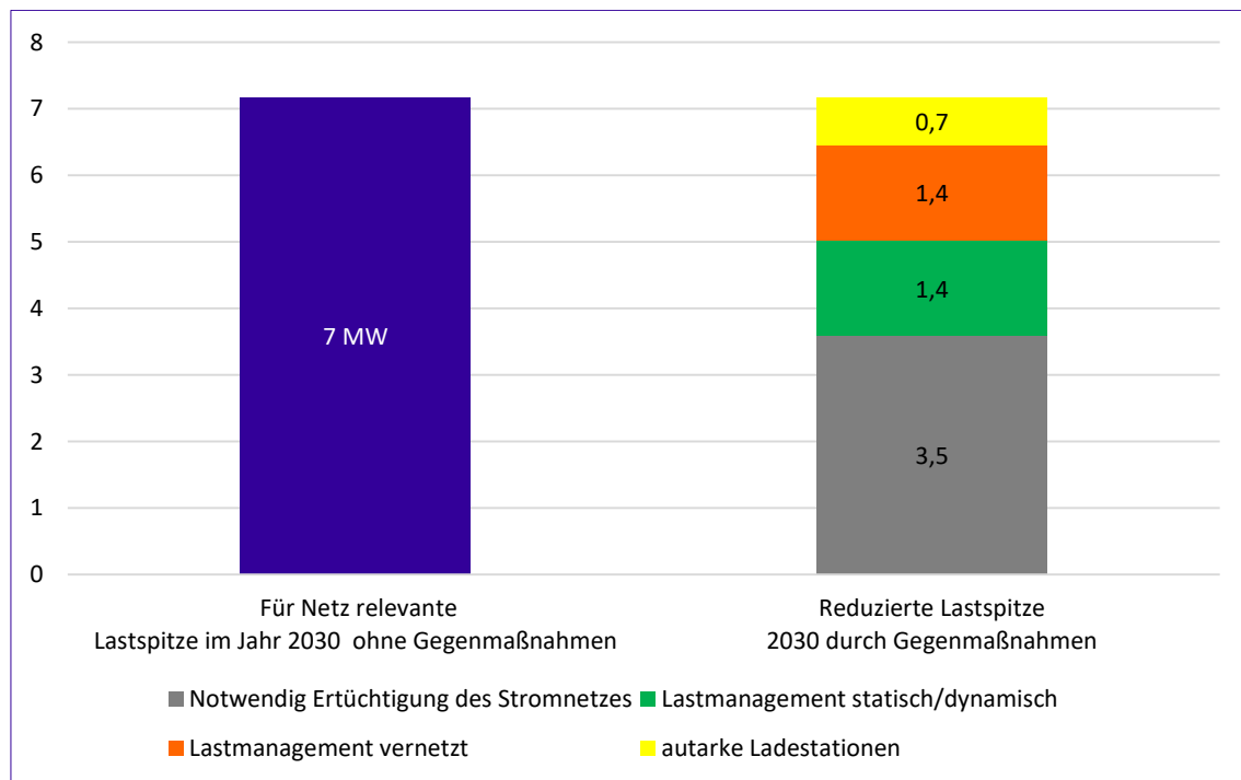
Abbildung 11: Reduzierte Lastspitze 2030 durch Gegenmaßnahmen (EIGENE BERECHNUNG 8 ).
