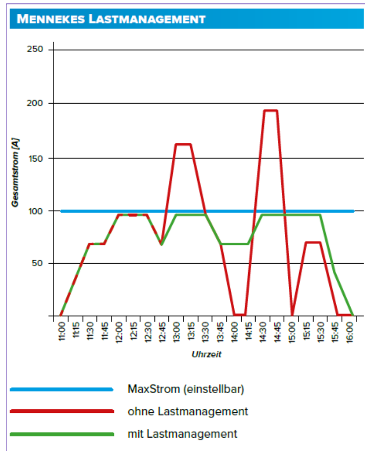
Abbildung 8: Lastmanagement (MENNEKES 2018).
