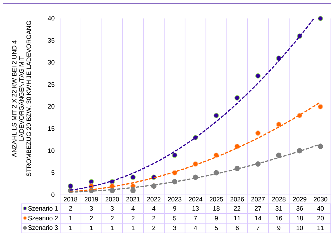
Abbildung 37: Anzahl der öfftl. benötigten Ladesäulen um den prognostizierten Strombedarf der E-Fahrzeuge im öfftl. Raum in 2030 zu decken. EIGENE DARSTELLUNG.
