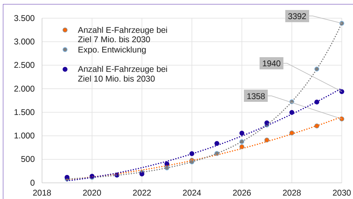
Abbildung 26: Prognostizierte Entwicklung der E-Fahrzeuge in Breisach. Eigene Berechnung. Datengrundlage KBA 2020A UND DIE BUNDESREGIERUNG 2020.
